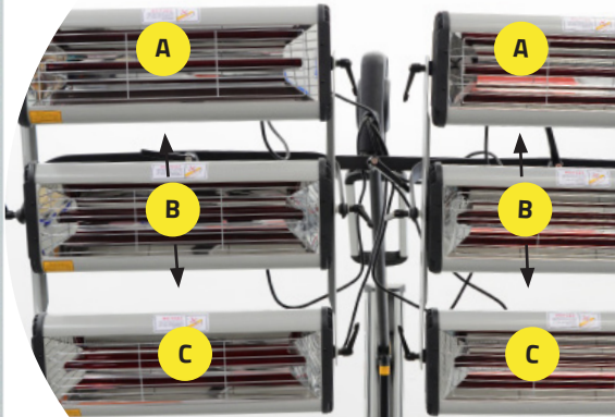
Le radiateur permet l'allumage des filaments dans n'importe quelle configuration : A+B+C, A+C, A+B, C+B, etc.
