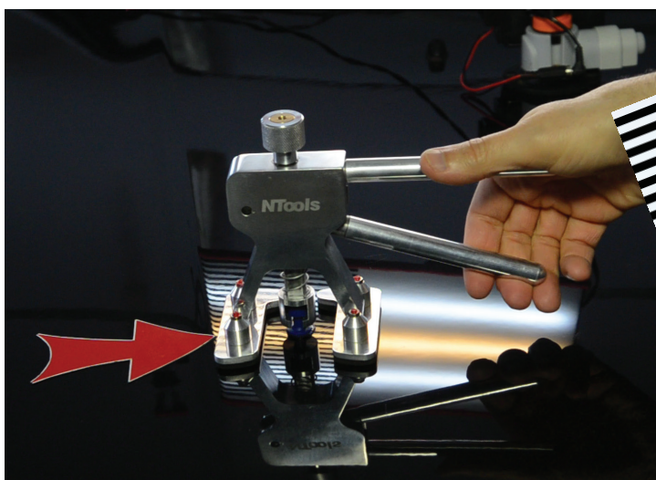
Lampa NTools PDR A12 z wkładką NTools WR przy pracy na naprawianym fragmencie karoserii.
