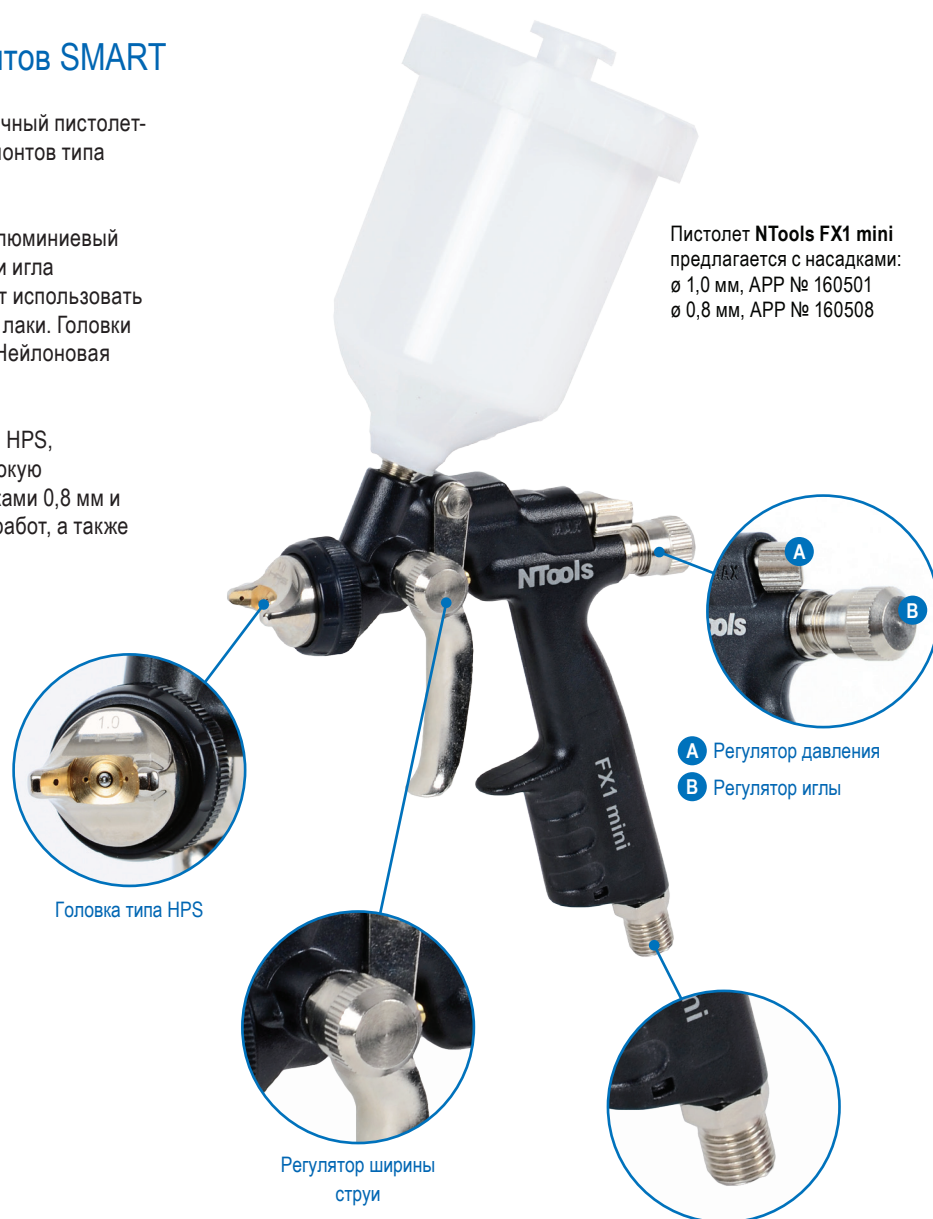
Резьбовое соединение 1/4"
